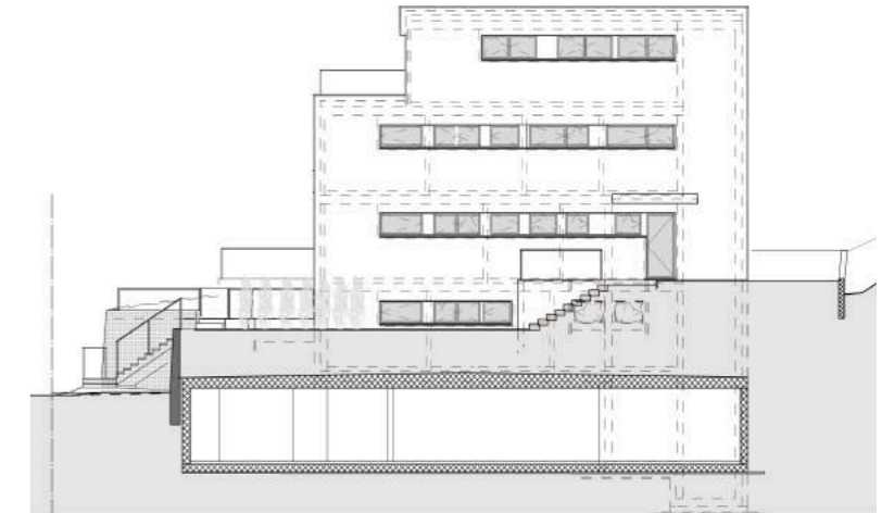
Nordwestfassade Haus 2
