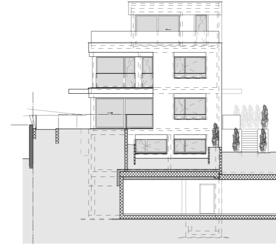
Nordostfassade Haus 2
