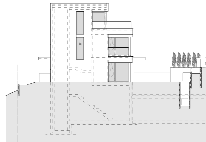
Südwestfassade Haus 1
