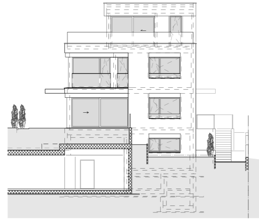
Nordostfassade Haus 1
