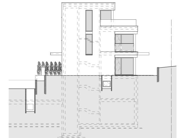
Südwestfassade Haus 2
