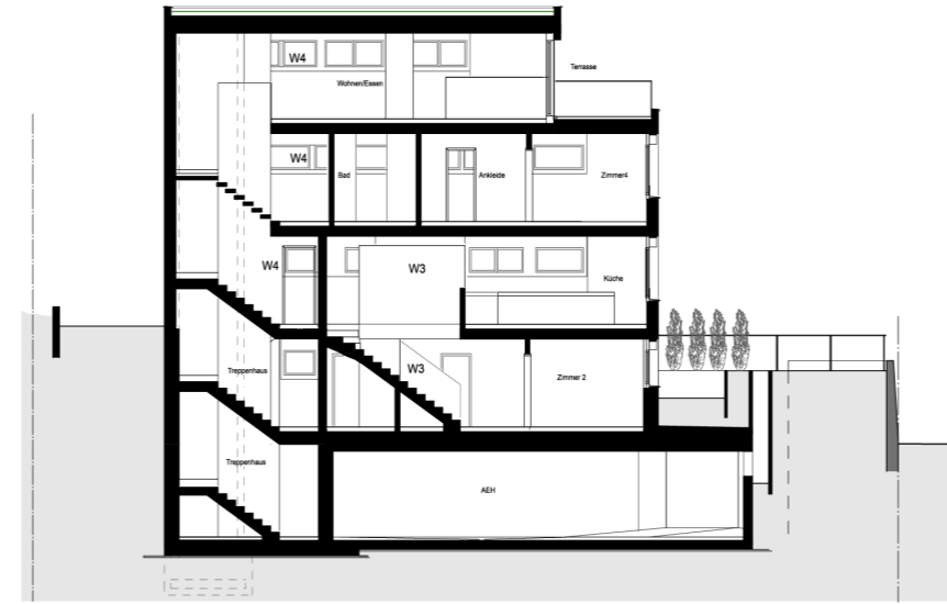
Schnitt 1 Haus 2
