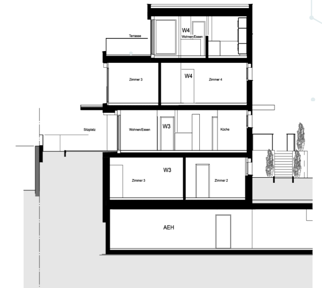
Schnitt 2 Haus 2
