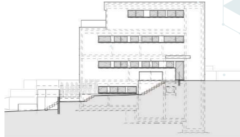
Nordwestfassade Haus 1
